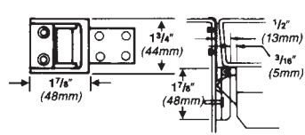
1439 Blade Stop
